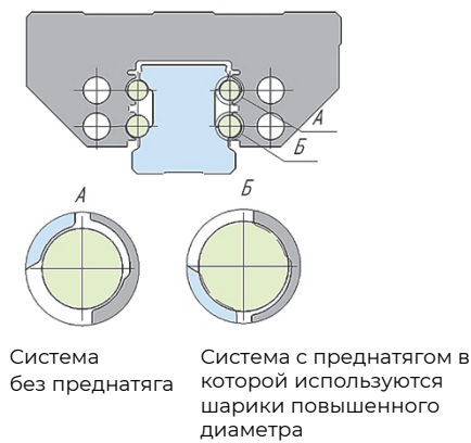
Создание преднатяга в роликовых системах реализуется по тому же принципу.
